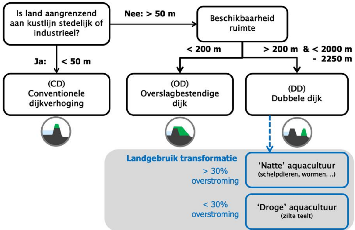
Figuur 3.2. Beslisboom voor implementatie van de drie inrichtingsscenario's. Voor DD wordt de volledige beslisboom doorlopen. Voor OD komt altijd bij >50 een overslagbestendige dijk, de dubbele dijk vervalt. In scenario CD komt altijd een dijkverhoging en vervallen opties voor overslagbestendige dijk en de dubbele dijk.
