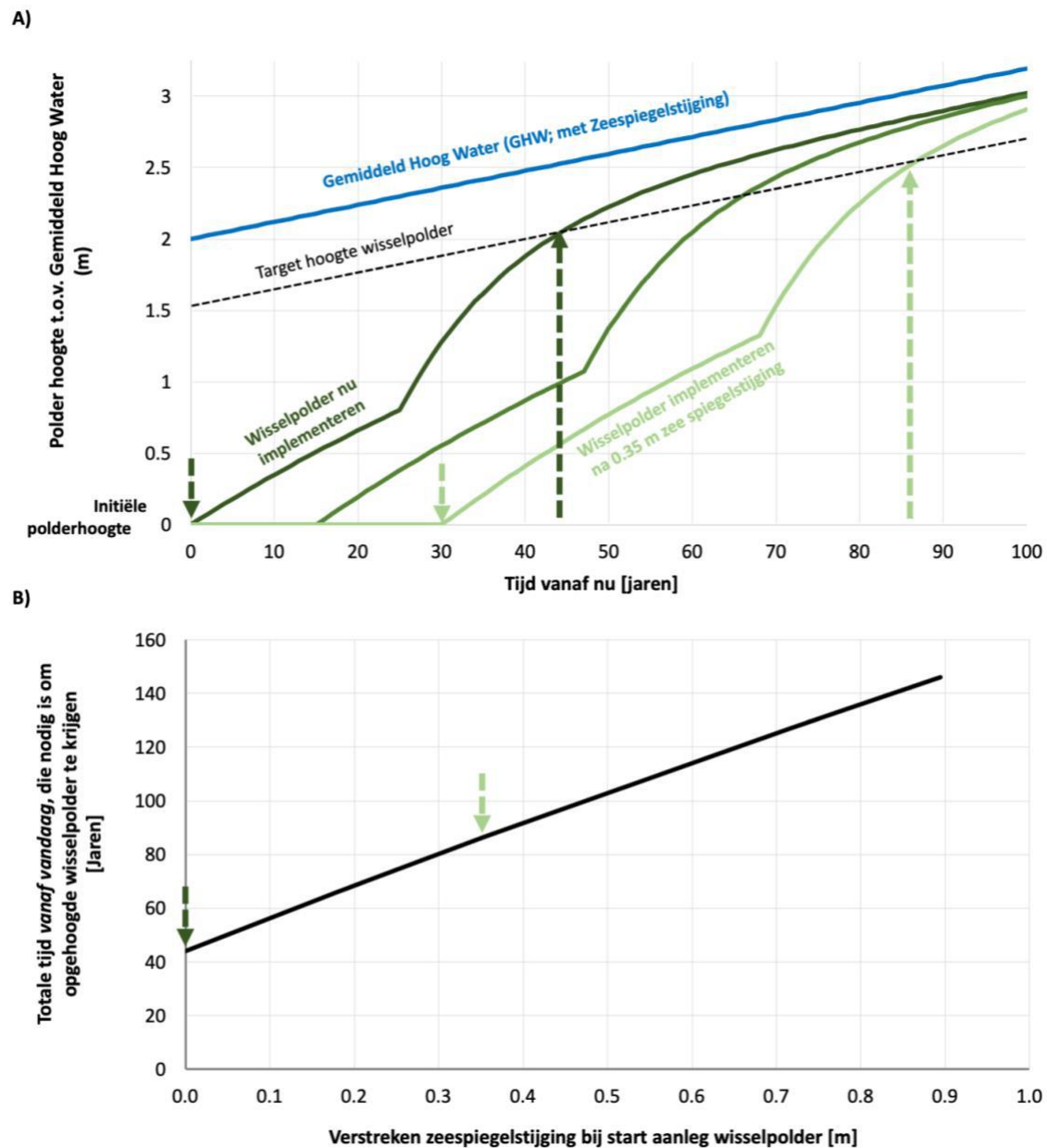
Figuur 3.7. Ontwikkeling van de bodemhoogte in de wisselpolder kost tijd. (A) wanneer direct wordt gestart dan kost het in een typische 30 – 50 jaar (in dit rekenvoorbeeld 44 jaar) om de gewenste hoogte te bereiken. Wordt de wisselpolder pas na 15 of 30 jaar geopend, dan heeft er meer relatieve zeespiegelstijging (incl. bodemdaling) plaatsgevonden waardoor het langer duurt om de gewenste bodemhoogte (target) te bereiken (respectivelijke 66 en 87 jaar). (B) Hoe langer zeespiegelstijging is voortgeschreden hoe langer er nodig is om de gewenste bodemhoogte te bereiken. De toename in benodigde extra tijd is 0,38 jaar per jaar uitstel wat overeenkomt met een extra 32 jaar tot target per 1 m relatieve zeespiegelstijging.
